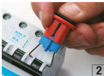
2 Pino para Dentro (Ponta Azul)
