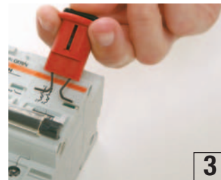
3 Pino para Fora Grande (Ponta Vermelha)
